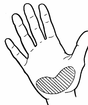
Figure 8.9 : Talon de la main
